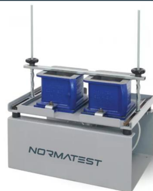
MESAS VIBRADORAS
